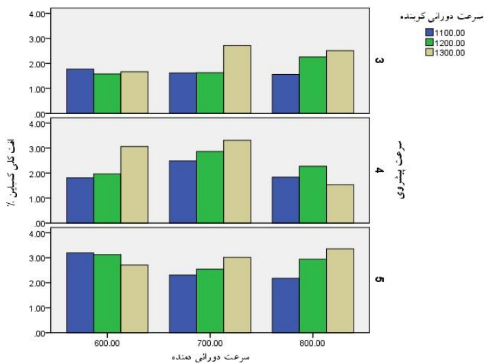
شکل ۵- میانگین درصد افت کلی کمباین در سطوح مختلف
