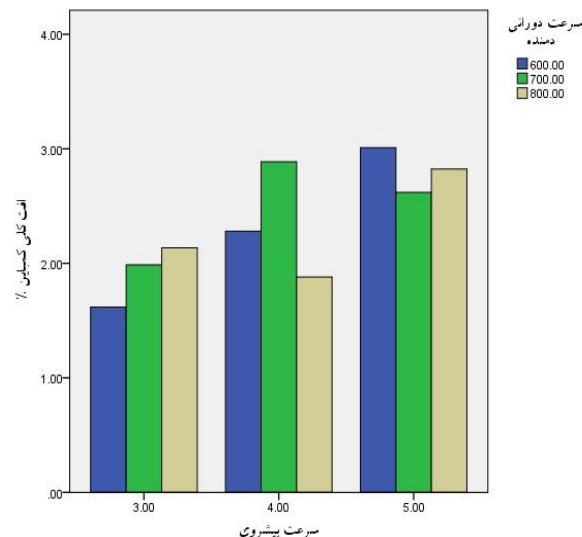
شکل ۴- اثر متقابل فاکتورهای سرعت پیشروی و سرعت دورانی دمنده بر درصد افت کمباین
