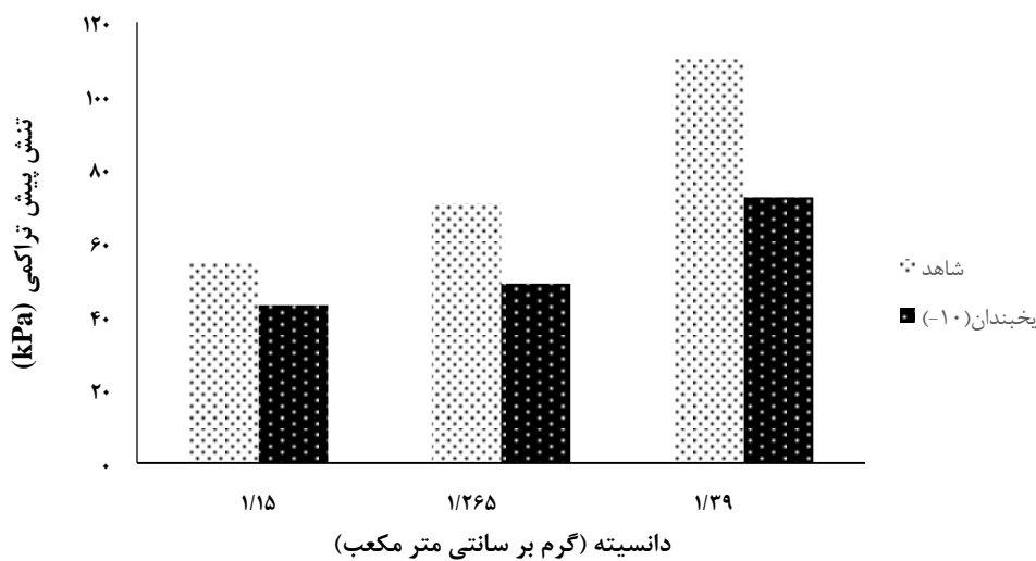
شکل ۴- نمودار تنش پیش تراکمی در رطوبت ۱۵ درصد
