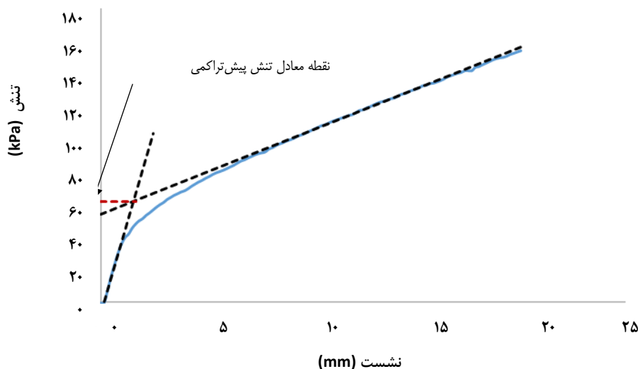
شکل ۲- محاسبه تنش پیش‌تراکمی به روش الکساندرو و ایرال
