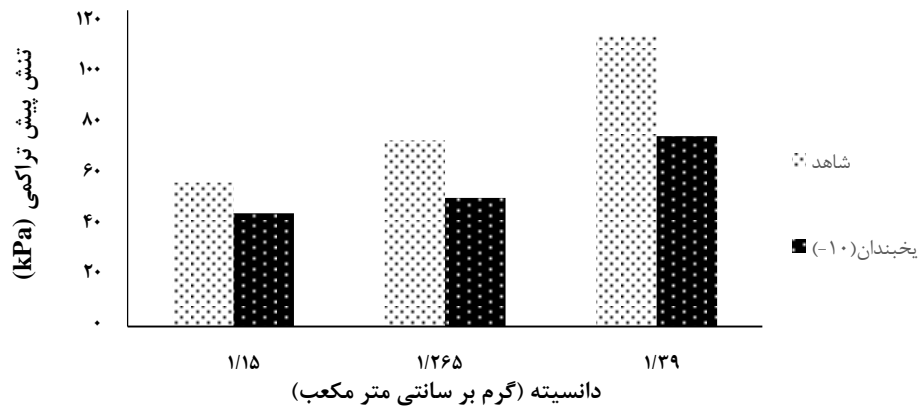
شکل ۳- نمودار تنش پیش تراکمی در رطوبت ۱۰ درصد
