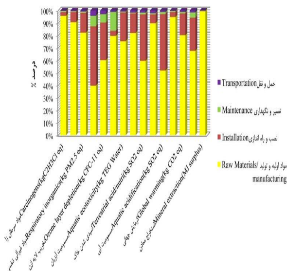
شکل ۲- سهم اثرات زیست محیطی در تولید الکتریسیته نیروگاه بادی آقکند در طول عمر ۲۰ سال
