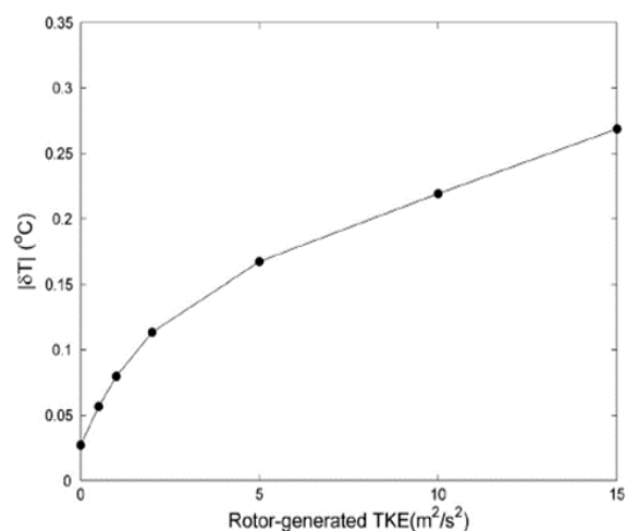
شکل ۵- تأثیر تلاطم بر مزارع بادی و تغییر دمای هوای نزدیک به سطح در مزرعه بادی
